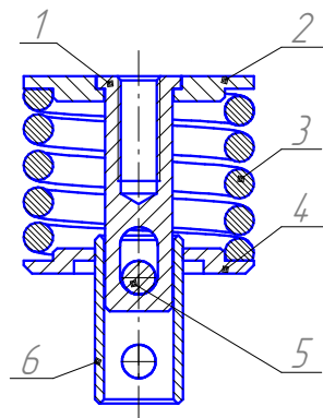
1,6- втулка; 2,4-шайба; 3- пружина; 5- ось; 6- втулка.
