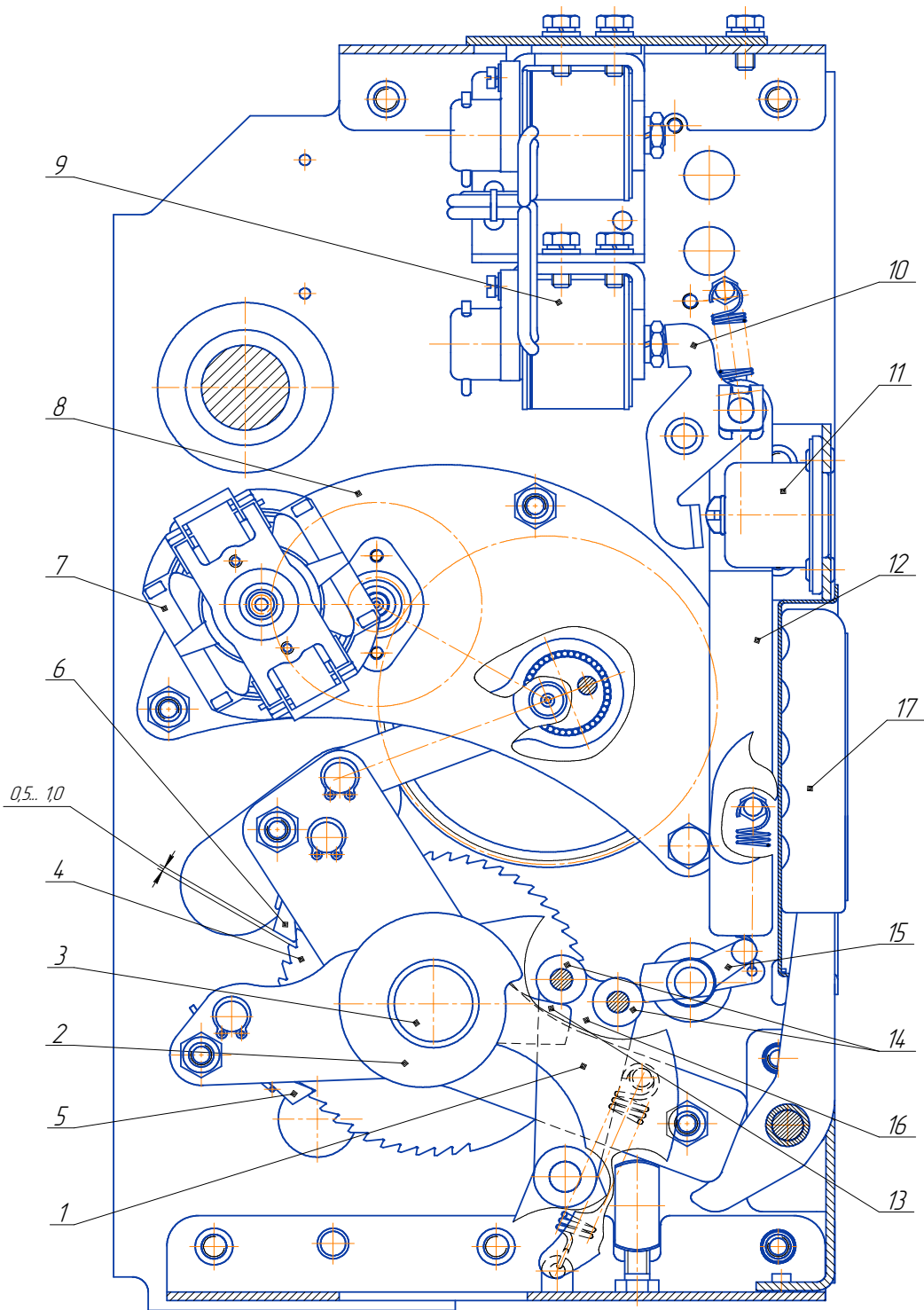
Рисунок 7 - Механизм привода
