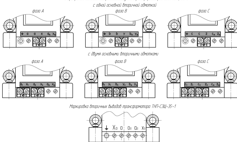
Маркировка выводов вторичных катушек трансформаторов НОЛ-СЭЦ-35-3
