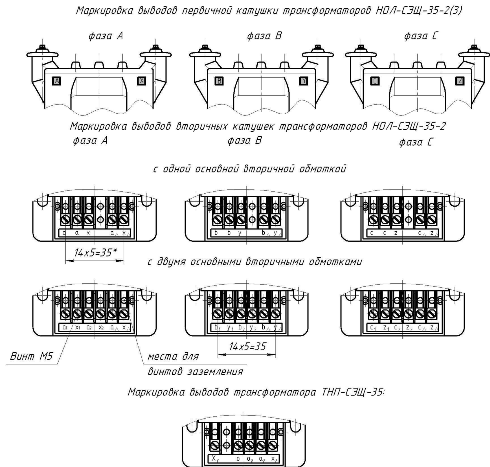
Рисунок 3 Маркировка выводов трансформаторов напряжения трехфазной группы НАЛИ-СЭЩ-35-1
