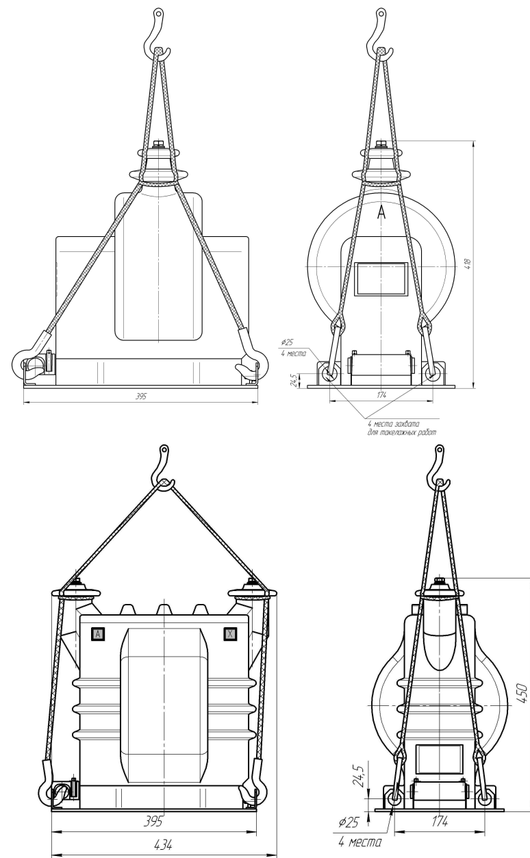
Рисунок 5 Строповка трансформаторов напряжения трехфазной группы НАЛИ-СЭЩ-35-1
