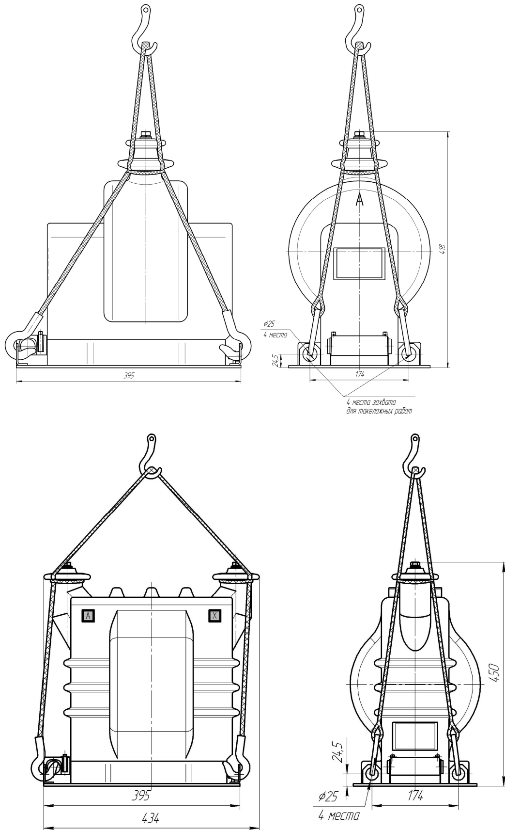
Рисунок 5 - Строповка трансформаторов напряжения трехфазной группы НАЛИ-СЭЦ-35-1
