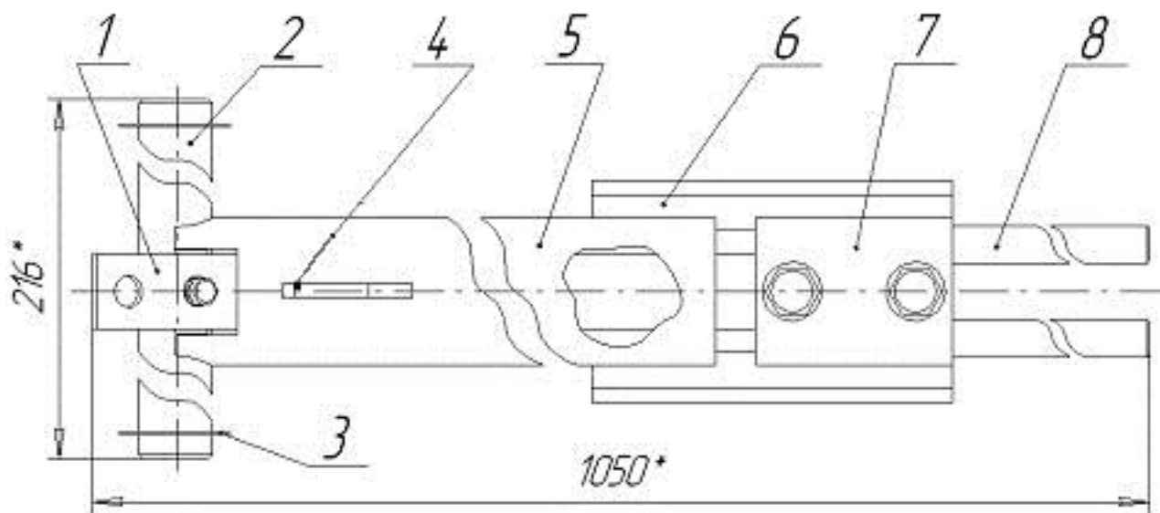
1 - шина; 2 - вал; 3 - стопорное кольцо; 4 - кронштейн; 5 - труба; 6 - направляющая скоба; 7 - прижимная скоба; 8 - ламель
