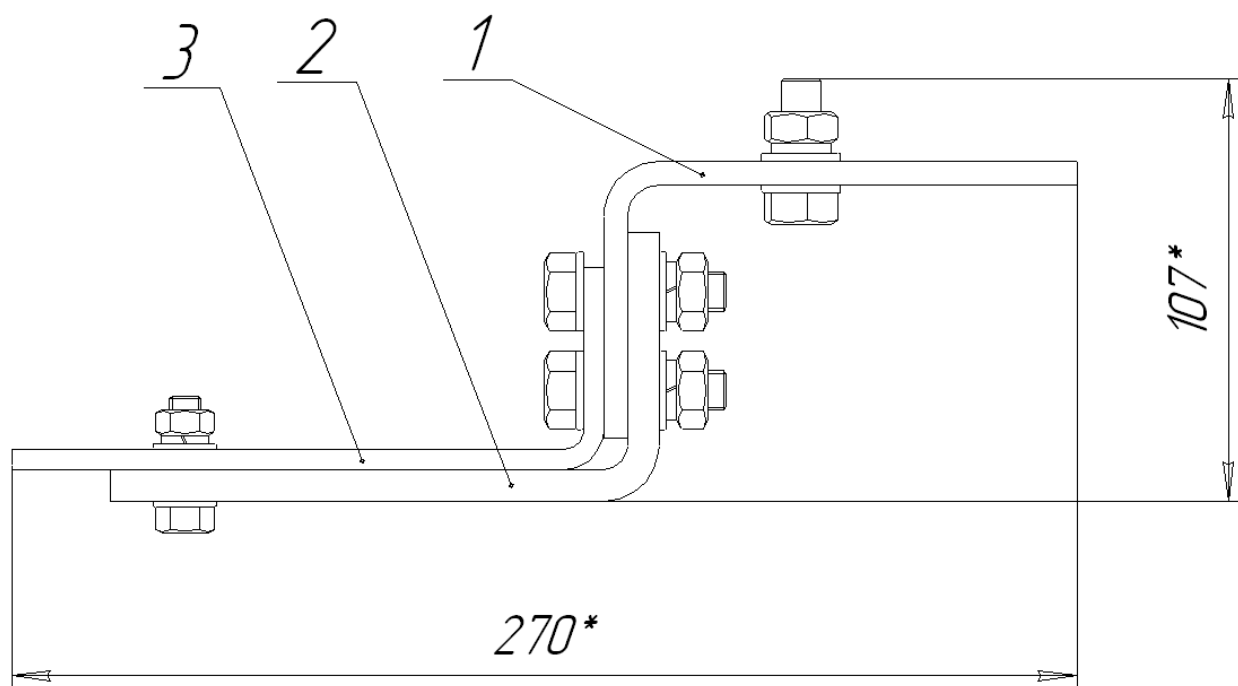
1 - верхний уголок ; 2 - контактодержатель; 3 - неподвижный контакт
