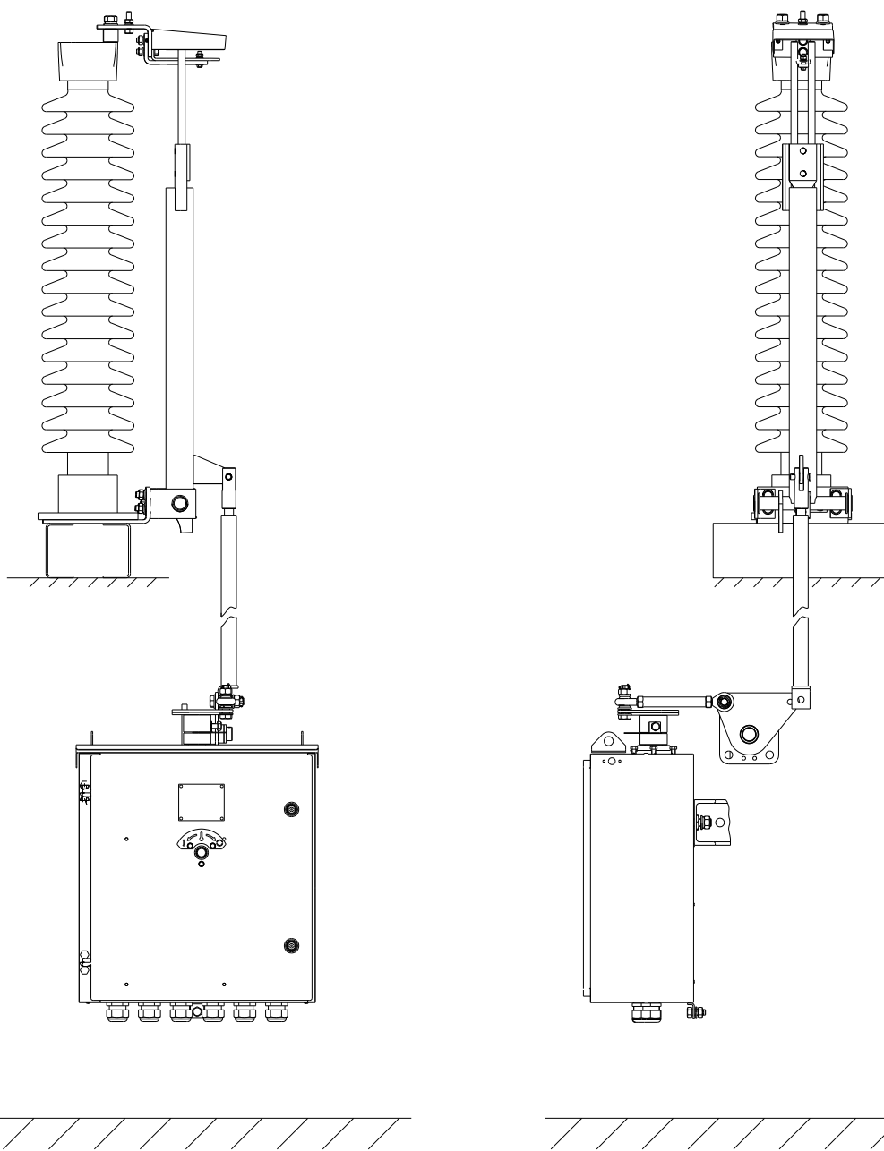
Рисунок А.5 – Заземлитель ЗОН СЭЦ® - 110-□/□ УХЛ1 с двигателем
